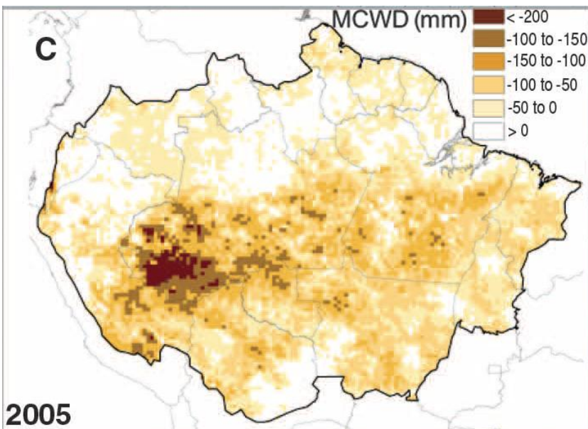
Lewis et al, 2011, Science
