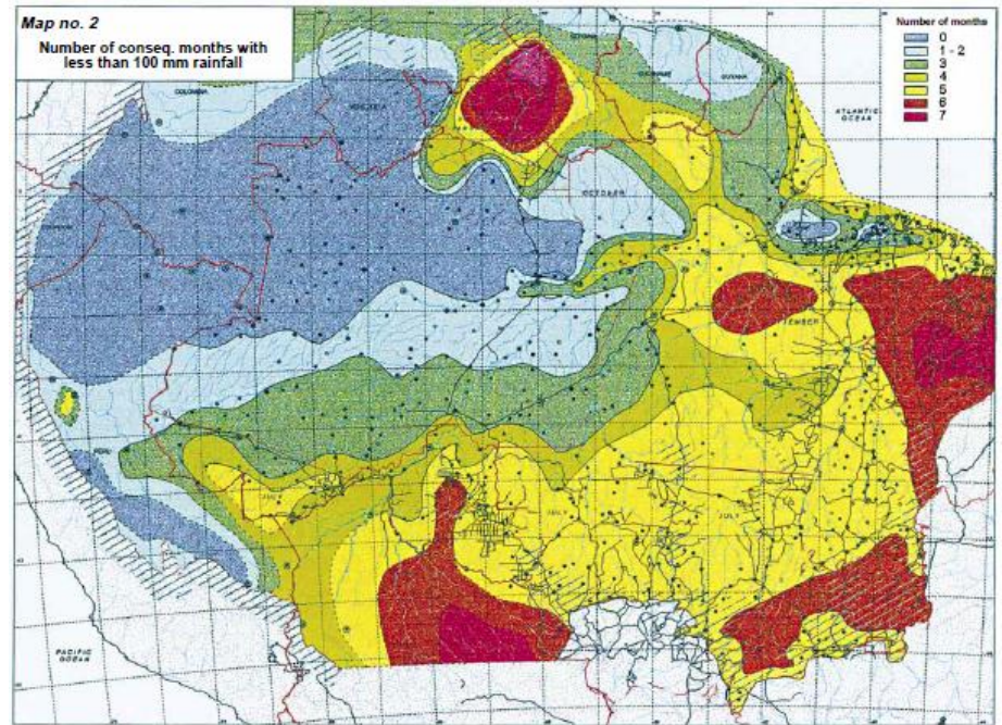
Sombroek, 2001, Ambio
